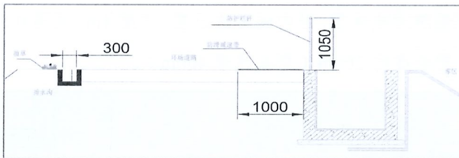
剖面图 2（陡坡段）
