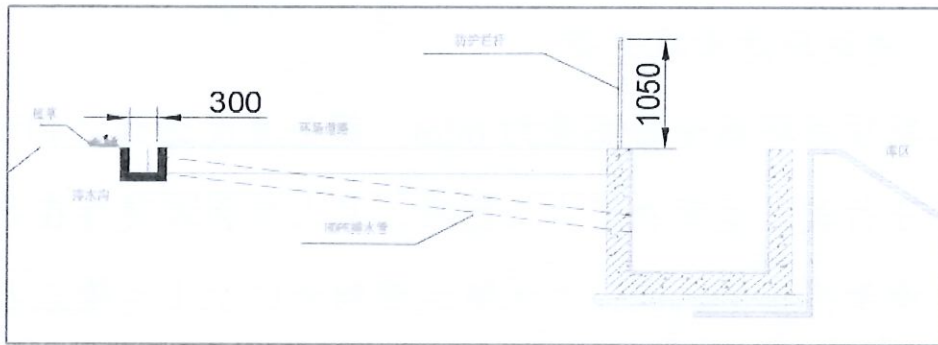
剖面图 1
